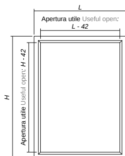
Vista fronte cassa senza porta Box front view without door
