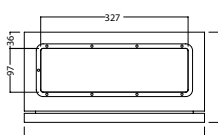
Vista pannello di cablaggio Wiring panel view
