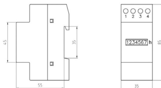
Din Rail Mount
